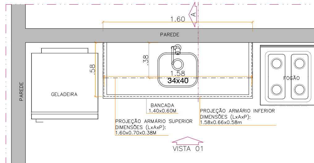
COPA - ARMÁRIOS 08,09 PLANTA BAIXA esc 1:25
