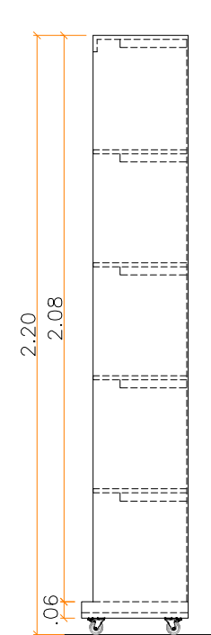
VISTA 02 esc 1:25
