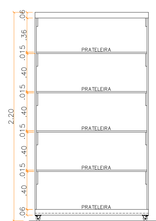
VISTA 01 esc 1:25
