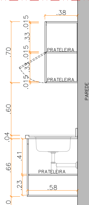
CORTE A - COZINHA ARMÁRIO 08,09 esc 1:25
