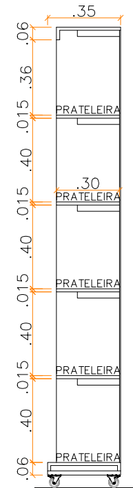
CORTE esc 1:25
