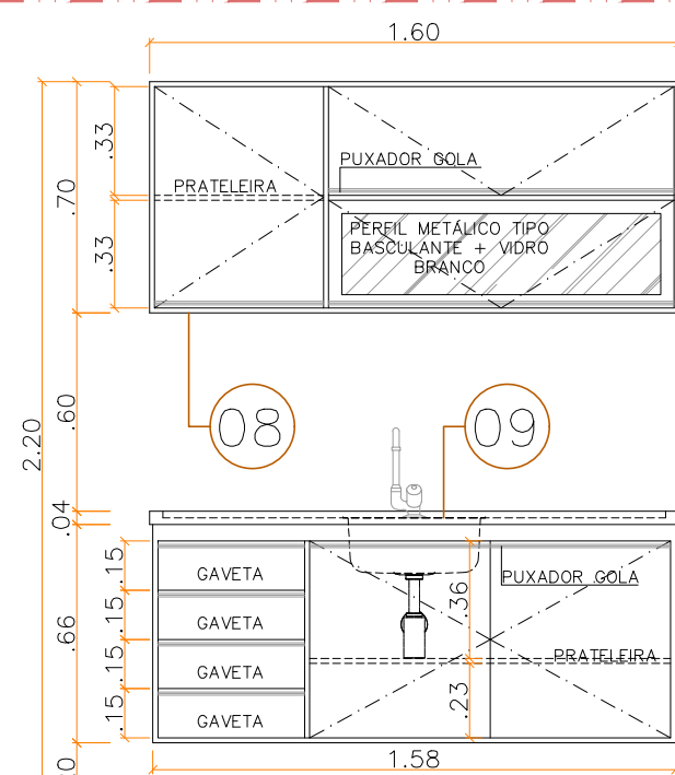
VISTA esc 1:25
