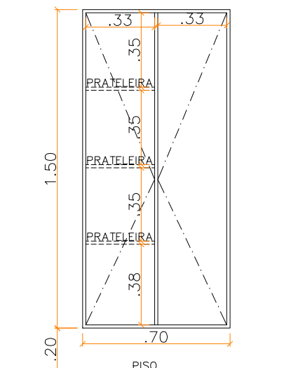
VISTA esc 1:25
